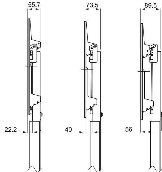
TV取り付け金具位置(S=1:10)
