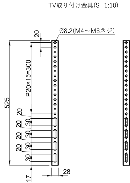
TV取り付け金具位置(S=1:10)
